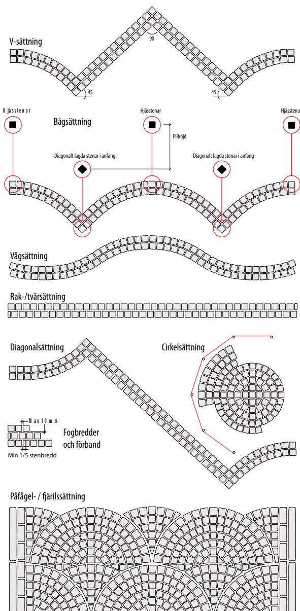
Fig 5.3 Principer för olika mönstersettingar med gatsten.
