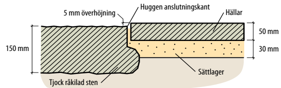
Fig 4.43 Anslutning av markbeläggning med hållar mot grov sten, t ex blocksteg eller kantsten.
