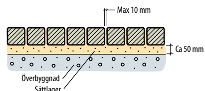
Fig 5.6 Typkonstruktion GS.
