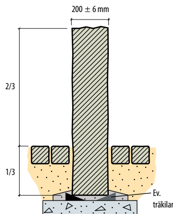
Fig 8.34 Montering av blockstensmur på betongplatta.
