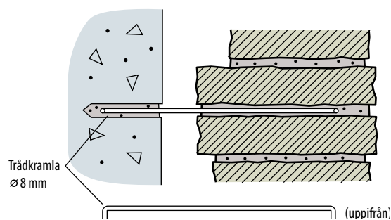
Fig 3.7 Hällarkramla av rundstång, ingjuten i betongstomme, monterad i fogar i mur av skivor
