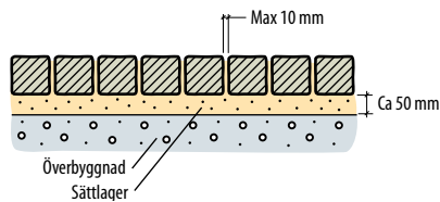
Fig 5.6 Typkonstruktion GS.
