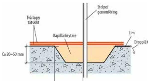
BILD 4. Diffusionsöppet cementbaserat tätskikt
