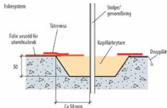
BILD 5. Diffusionsöppet cementbaserat tätskikt med nät
