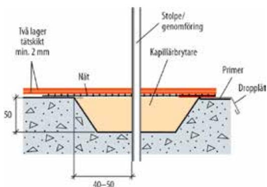
BILD 6. Foliesystem avsett för utomhusbruk
