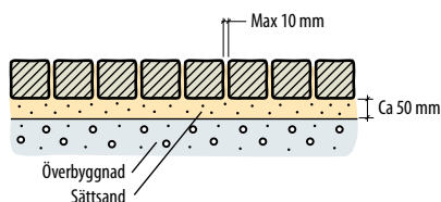
Fig 5.5 Typkonstruktion GS.
