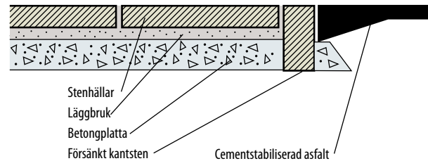
Fig 4.27 Konstruktion vid inläggning av hållar som markeringsband i asfalt.
