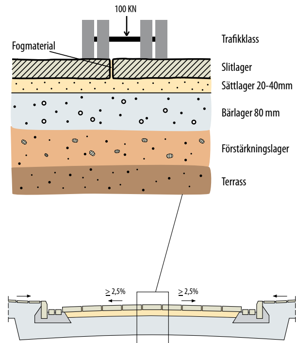
Fig 4.32 Uppbyggnad av vägbanan belagd med hällar. Kantsten som motstöd.
