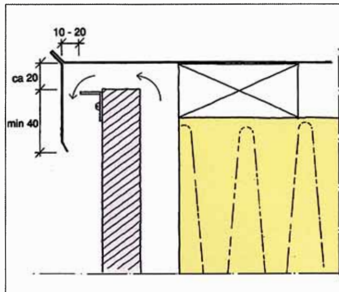
31. Luftutsläpp vid takfot i utsatt läge. List på stenen förhindrar vatten att driva över plattkanten.
