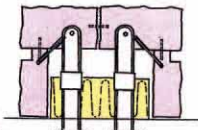
Horizontalsnitt, bäring
