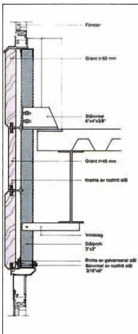
64. 40 resp 60 mm tjock granit monterad mot stålramverk av tunnplåtprofiler. Ramfackverken, som är ca 7 x 1,5 m, monteras mot byggnaden med speciella bärkonsoler i våningsplanen, kompletterade med stag för att motverka vindlast. Fasaden består av bröstnings- och pelarelement.
