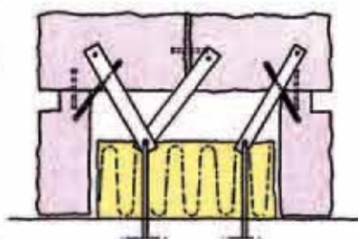
Horizontalsnitt, inhållning
