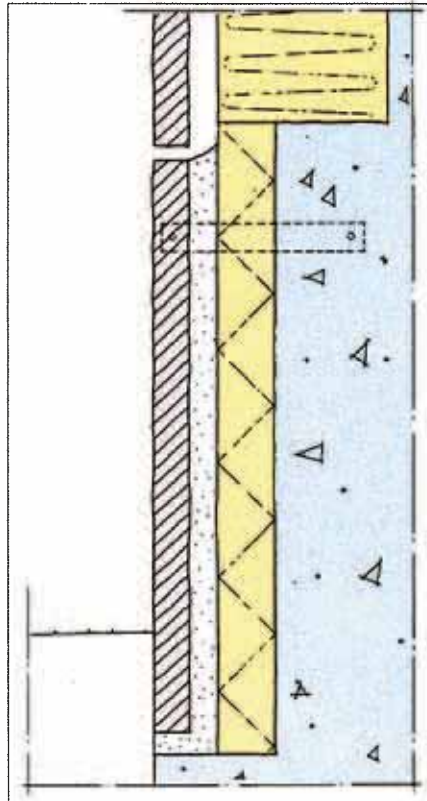
36. Bakgjuten sockel.
