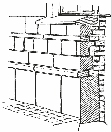
2. Fasadstenen murad som en integrerad del av byggnadens bärande stomme.
