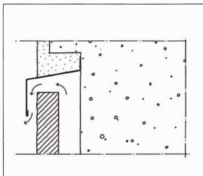
33. Plåtavtäckning skyddar luftutsläppet i anslutning mot annat fasadmateriel (puts).
