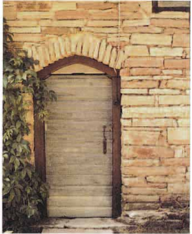
1. De första naturstensfasaderna byggdes av staplade block och hällar. Kantställda skivor bildar valv över öppningar.
