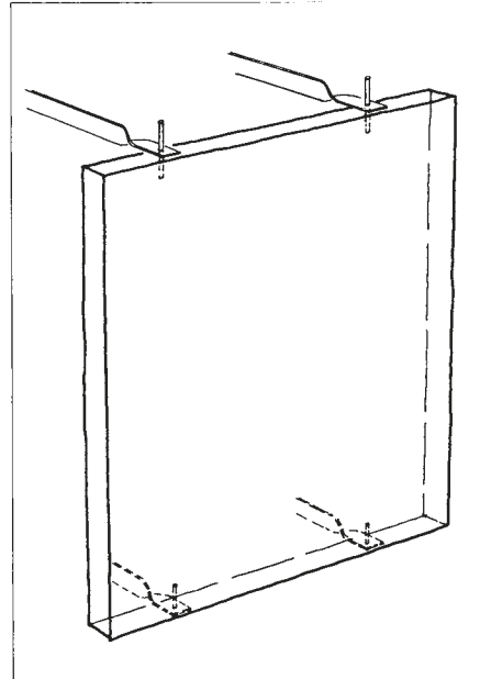
7. Platta monterad med Bh-kramlor i horisontal- (ligg-) fogarna, underkramling.
