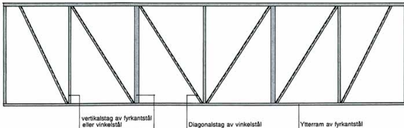
62. Exempel på utformning av ramfackverk för naturstensbeklädnad.
