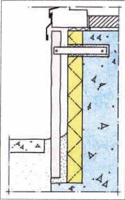
70. För att minska risken för intryckning bör ej gångbanebeläggningen läggas direkt mot sockeln.
