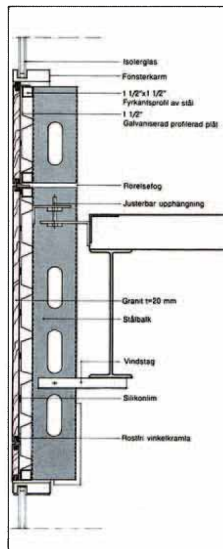
65. Lättvikts-element klädda med endast ca 20 mm (3/4") tjock granit. Ramverket är uppbyggt av balkar av galvaniserat stål. På utsidan har monterats en trapetsprofilerad plåt och ytterst granitplattorna. Naturstenen bärs av en kombination av kramlor av rostfritt stål och silikonlim. Denna metod innebär större möjligheter för elementet att ta upp rörelser, bl a som följd av vindlast.
