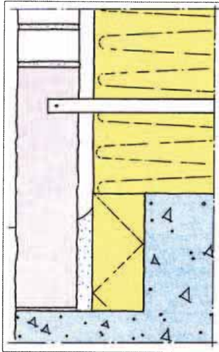
71. Sockel av tjock sten är tålig mot mekanisk åverkan. Den kan även dimensioneras för att bära ovanliggande fasadmaterial, t ex tegel.
