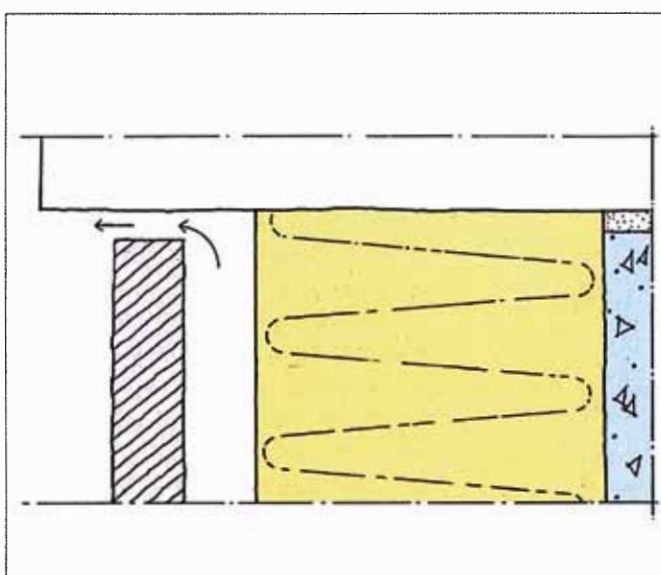
32. Luftutsläpp mot annat fasadmateriel, som skyddar mot vatteninträngning. Öppningar kan alternativt göras i stötfogarna.
